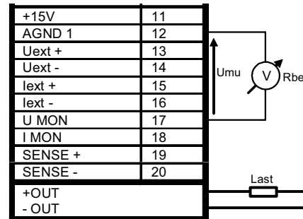
Bild 7.6 Verdrahtung Spannungsmonitor.
