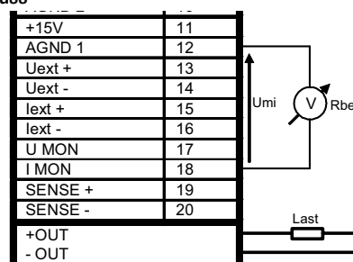
Bild 7.7 Verdrahtung Strommonitor.
